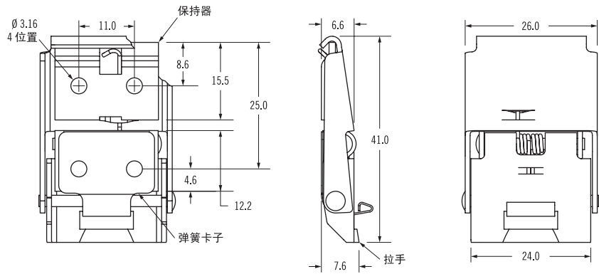
图示为弹簧型
