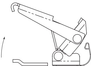
松开拉手 及开启门锁弹簧
